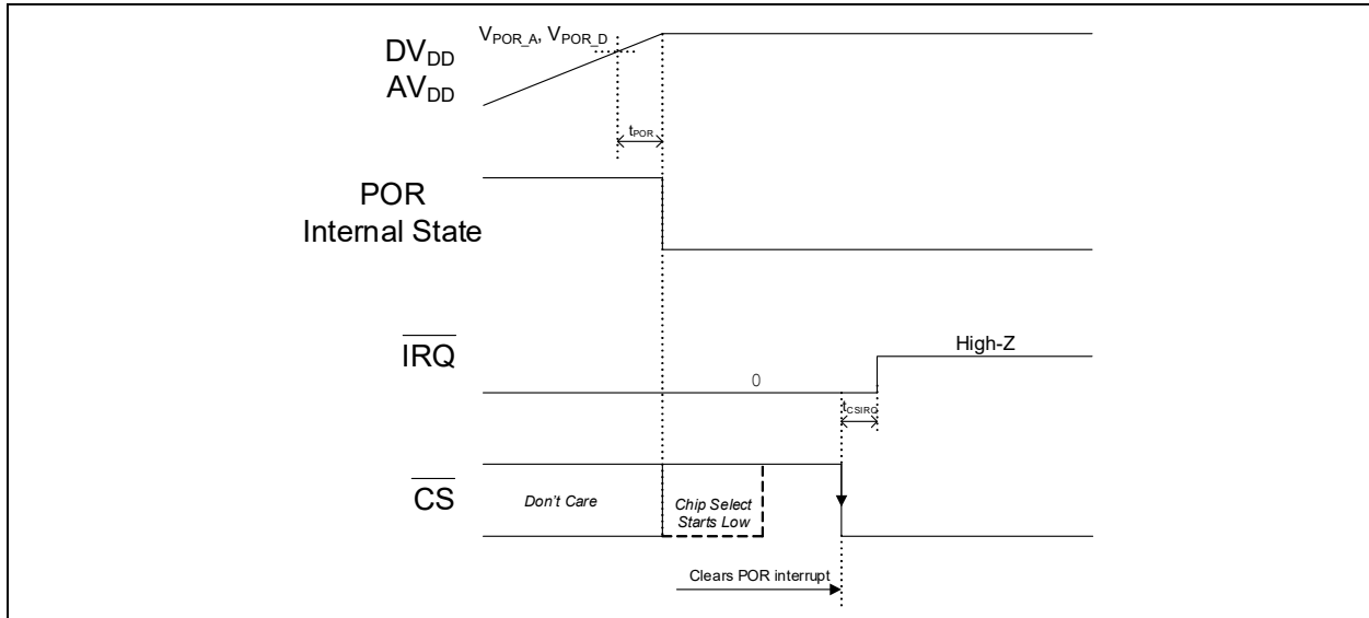
FIGURE 6-15: POR \overline{IRQ} Timing Diagram.
