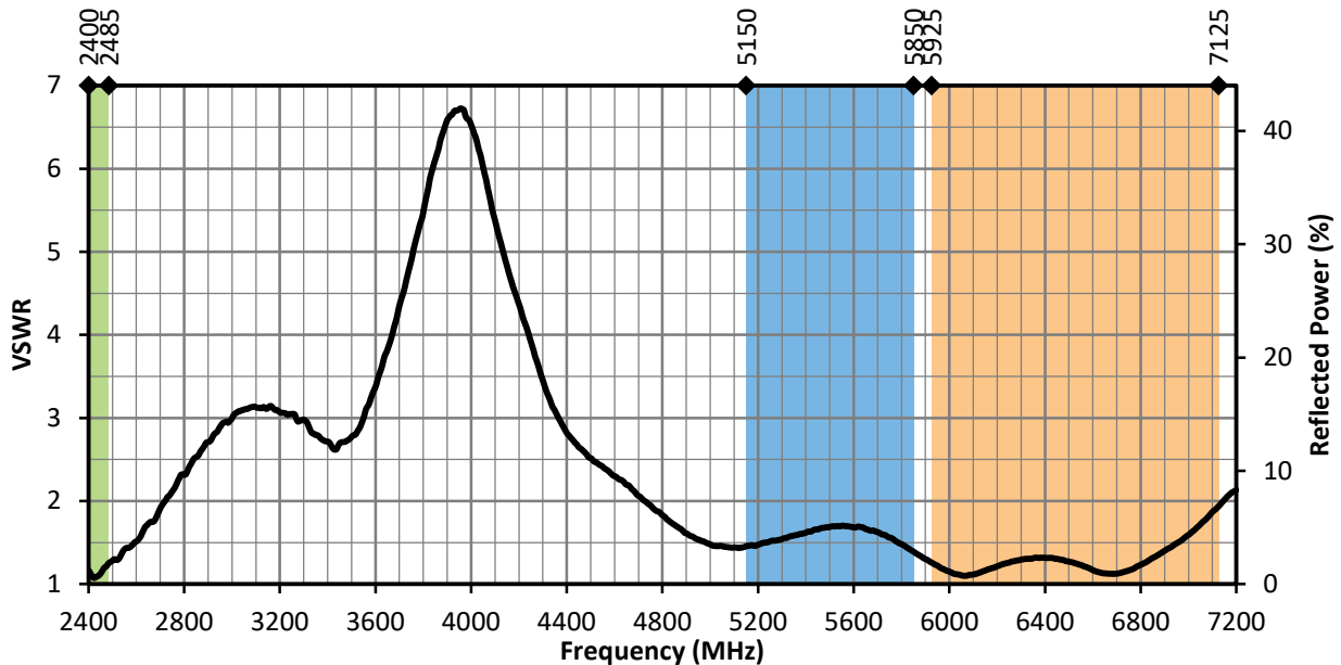
Figure 11. ANT-W63WS4-ccc VSWR, Edge-Bent
