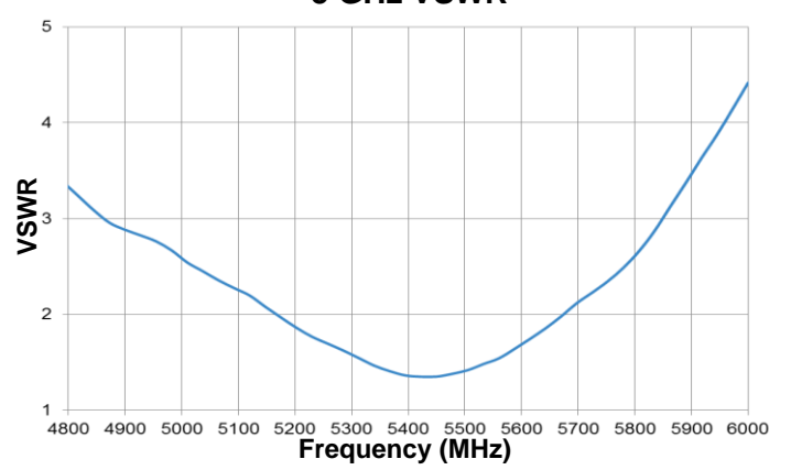
5 GHz VSWR
