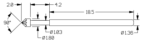
P25-5223 Star Head
